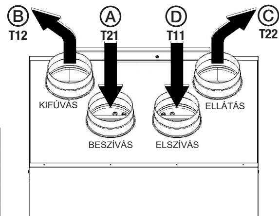
7.b ábra QR400A és QR550A hőmérsékleti érzékelői.
