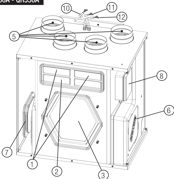
8.b ábra QR400A és QR550A belső alkatrészek
