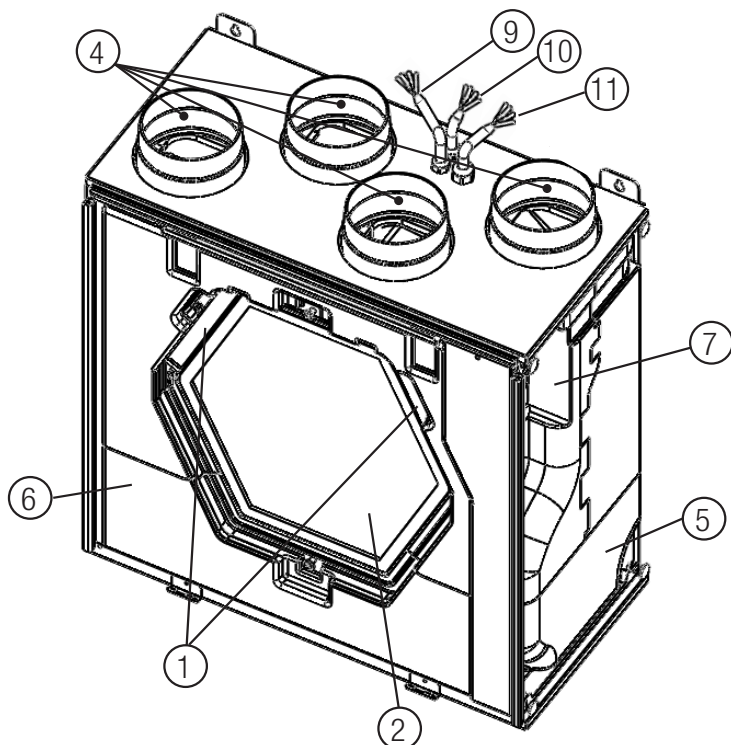
8.a ábra QR280A belső alkatrészek
