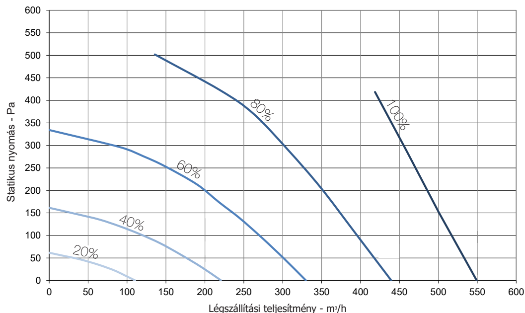
6.e ábra Bemeneti görbe az 1253/2014/EU (ErP) rendelet szerint. A termék tesztelése F7 típusú szűrő nélkül történt.
