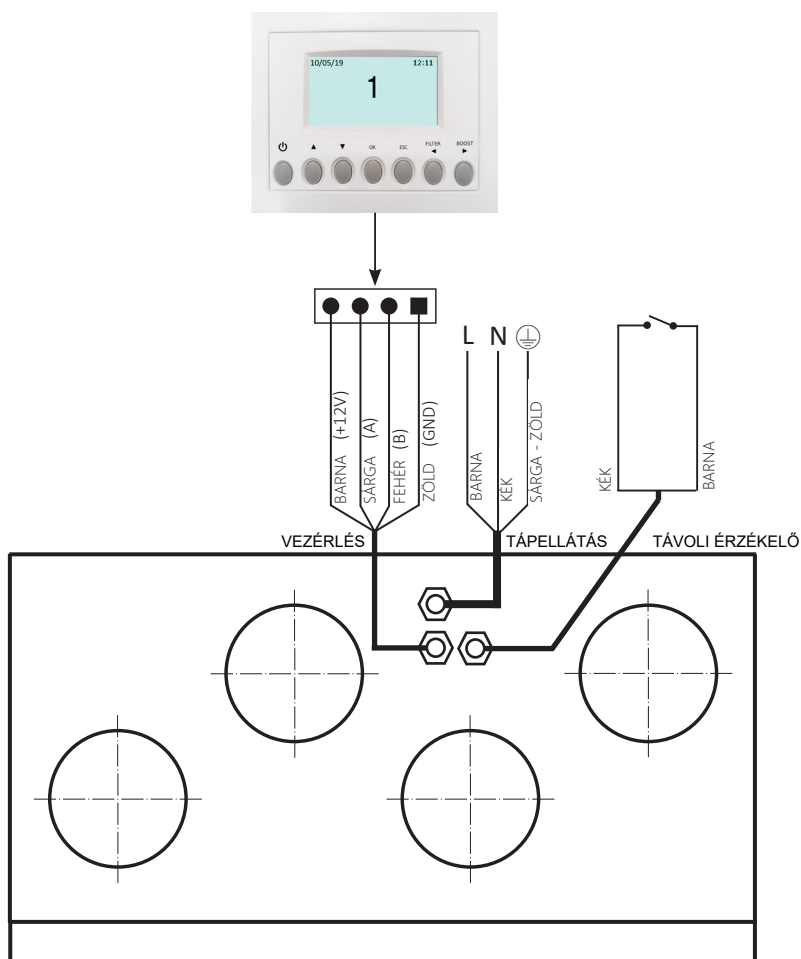
5.p ábra Elektromos csatlakozások
