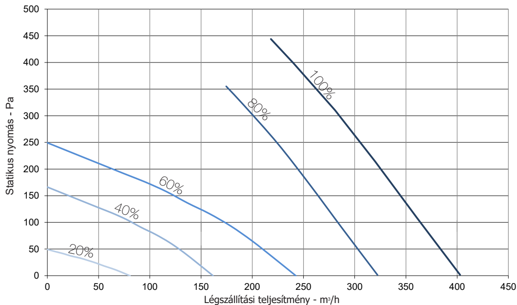
6.c ábra Bemeneti görbe az 1253/2014/EU (ErP) rendelet szerint. A termék tesztelése F7 típusú szűrő nélkül történt.
