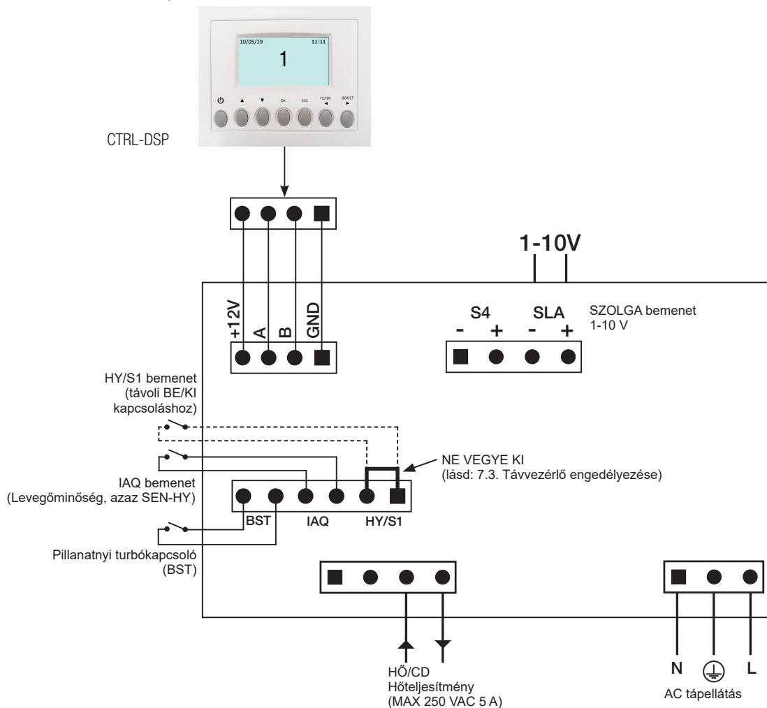
5.q ábra Elektromos csatlakozások a csatlakozódobozba szerelt alaplapon
