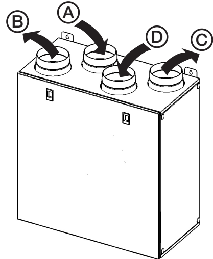
3.a ábra Csatlakozások BAL és JOBB oldali irányban - QR280A.
