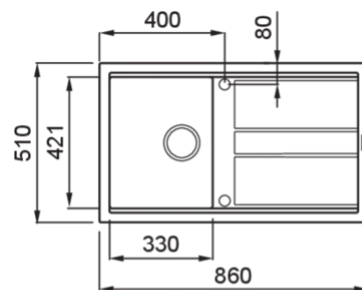
Méretrajz
