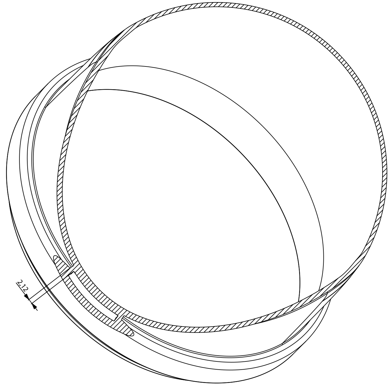
SEZIONE D-D
