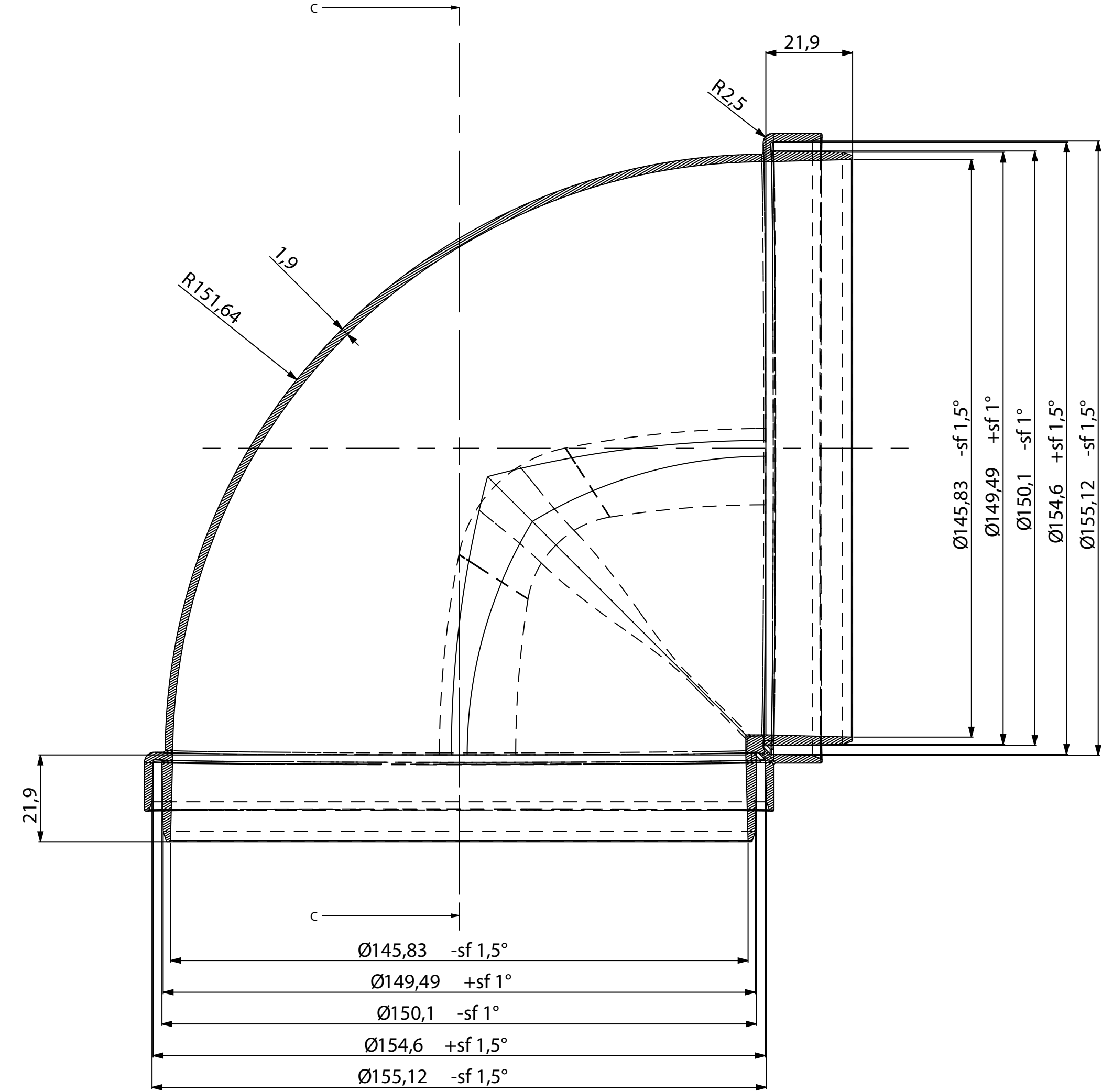
SEZIONE A-A
