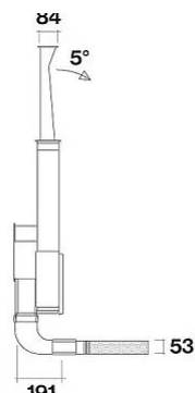
Oldalnézetben történő beépítés Slim motorral hátul, KACL.951 aljzatszűrővel (h 60mm)
