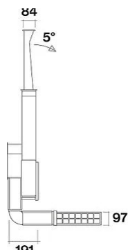
Oldalnézetből történő beépítés Slim motor hátuljával
