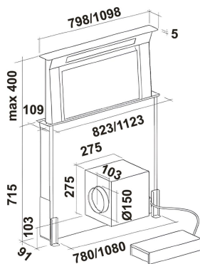
Szívó kivitel (motor 950 m 3 /h motorral a motorháztetőre szerelve)
