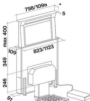
Szűrős változat (Slim motor) Carbon.Zeo szűrővel alatta (KACL.930)
