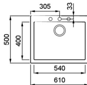
Méretrajz
