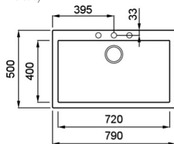
Méretrajz
