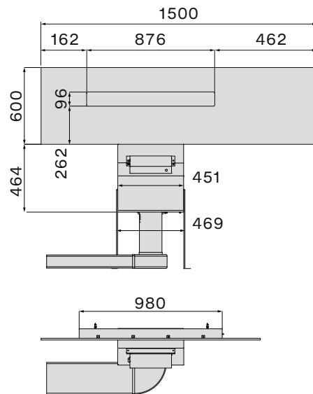
előlnézet 150 cm-es modul bal oldali elszívással
