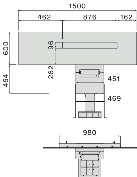
Szűrős változat - előlnézet 150 cm-es modul jobb oldali elszívással
